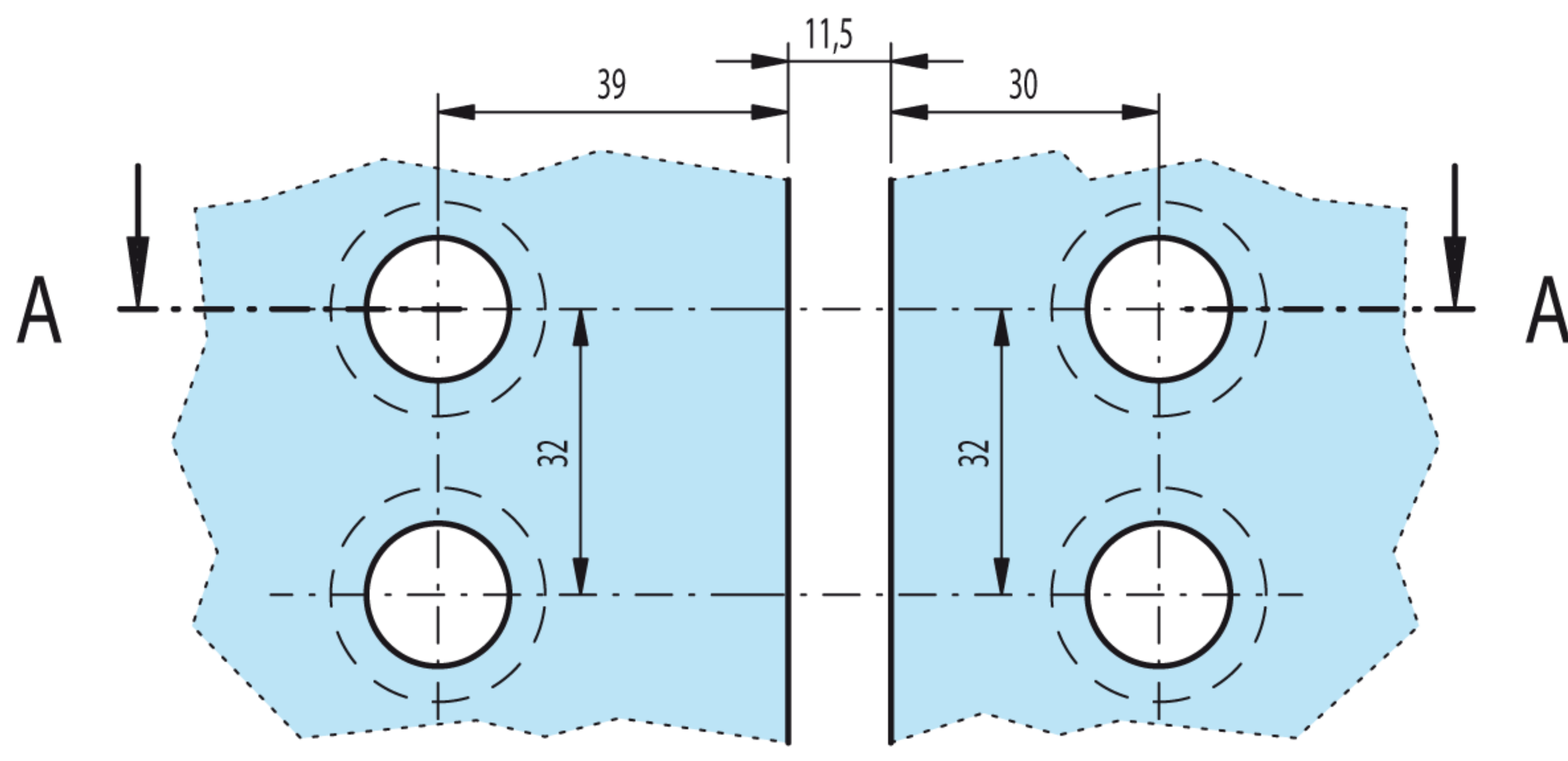
Festteilglas 2
