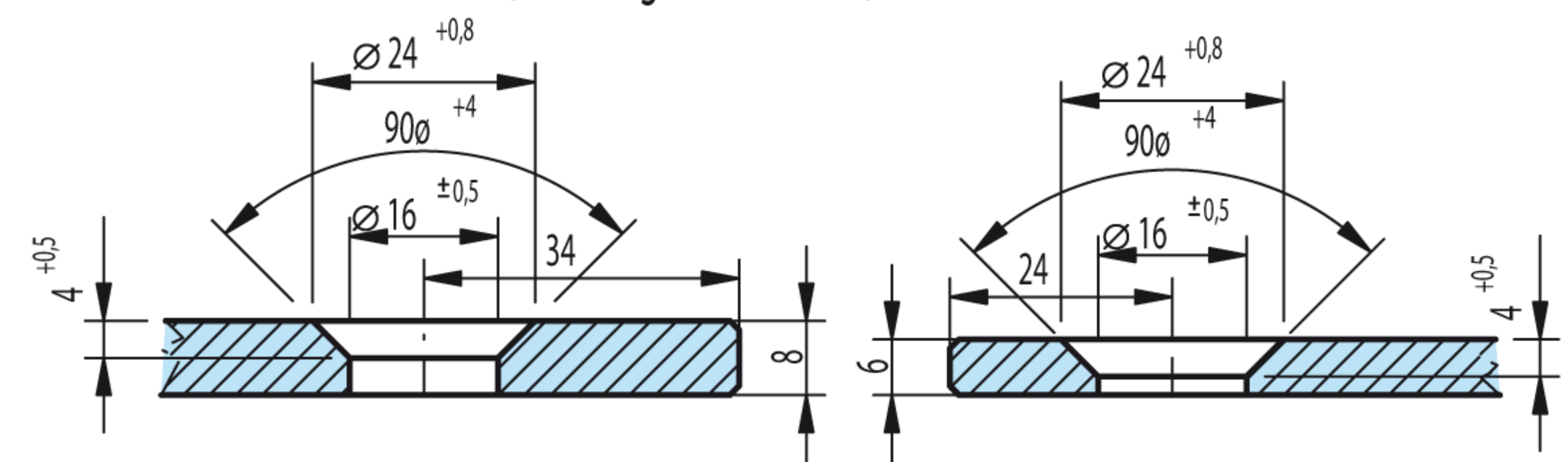
Schnitt: A-A (M1:1)
