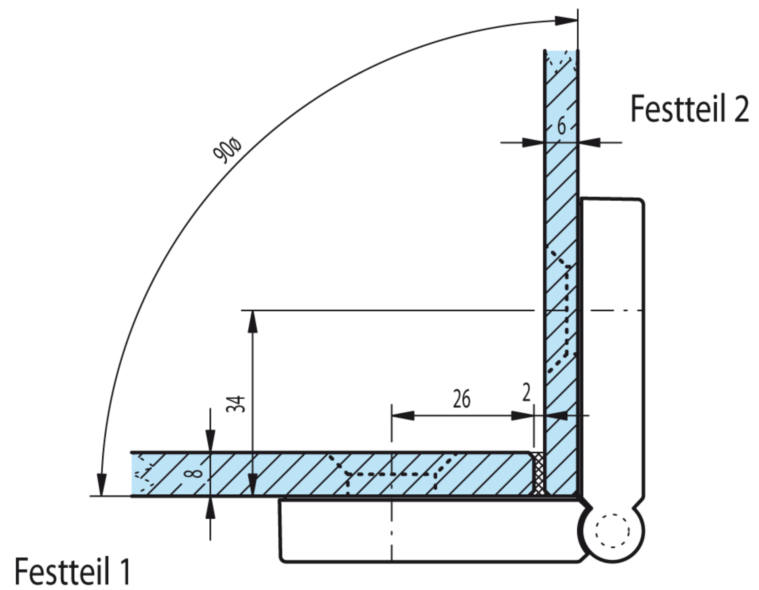
Schnitt: A-A (M1:1)
