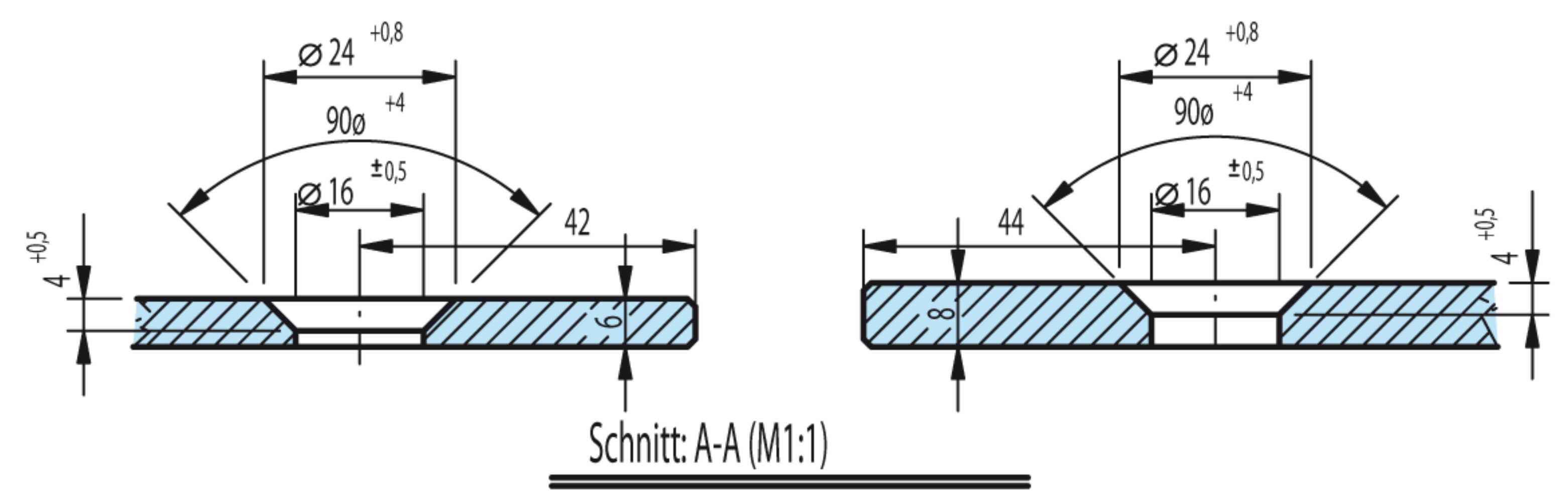
Flügelglas (Senkung = Innenseite) Festteilglas
