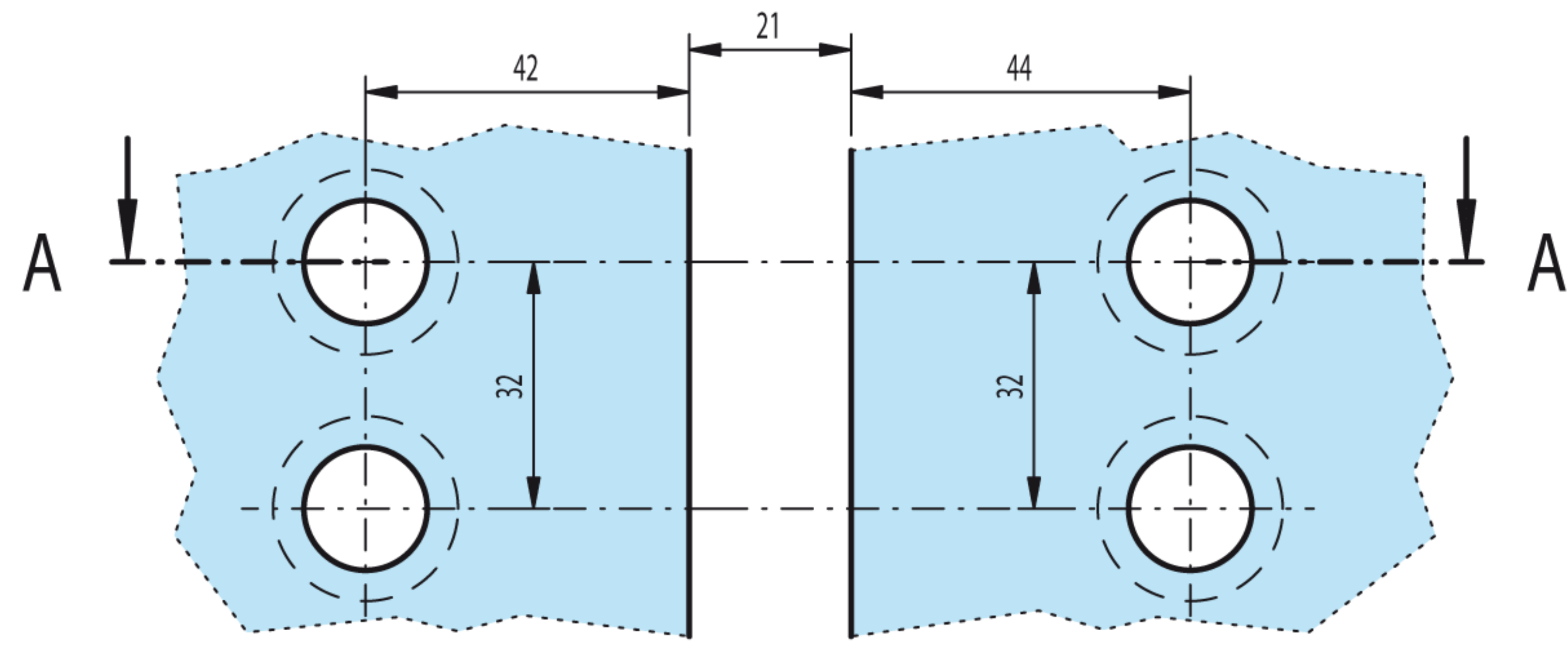
Flügelglas (Senkung = Innenseite) Festteilglas
