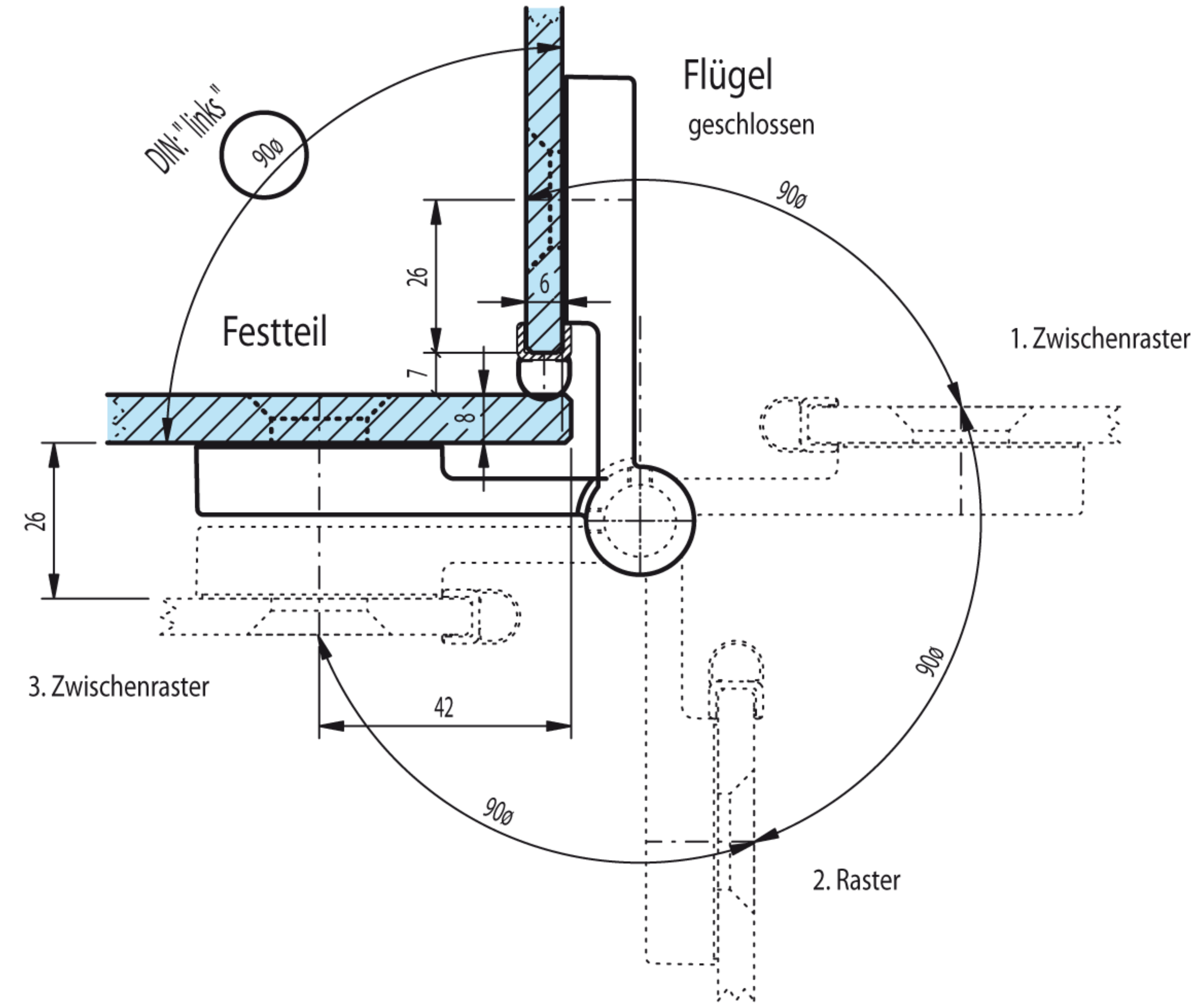
Schnitt: A-A (M1:1)
